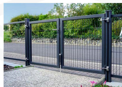
Tor Kombination und Rahmen mit eingepasster Stabmatte
